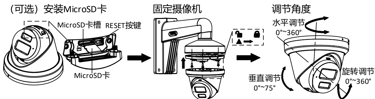
图1-6 壁装 (1)
