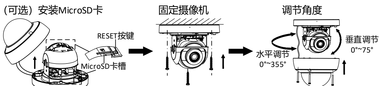
图1-9 吸顶装
