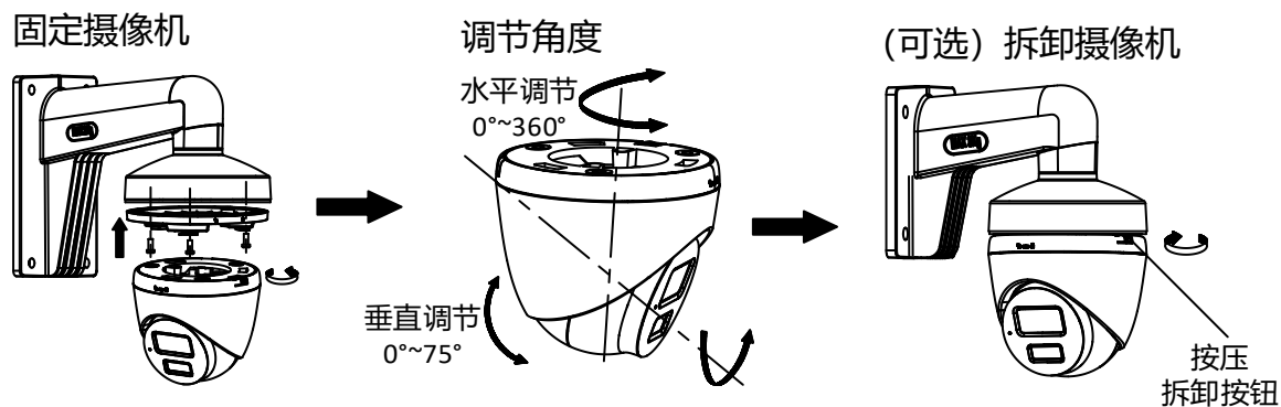
图1-7 壁装 (2)
