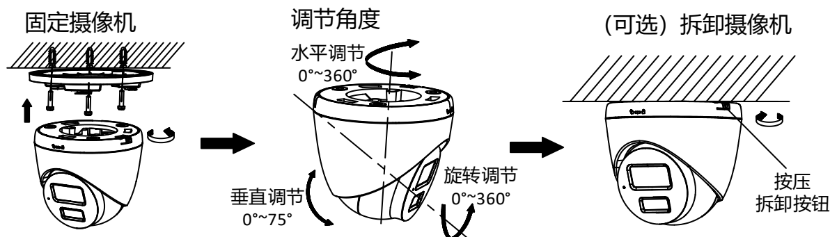
图1-5 吸顶装 (2)
