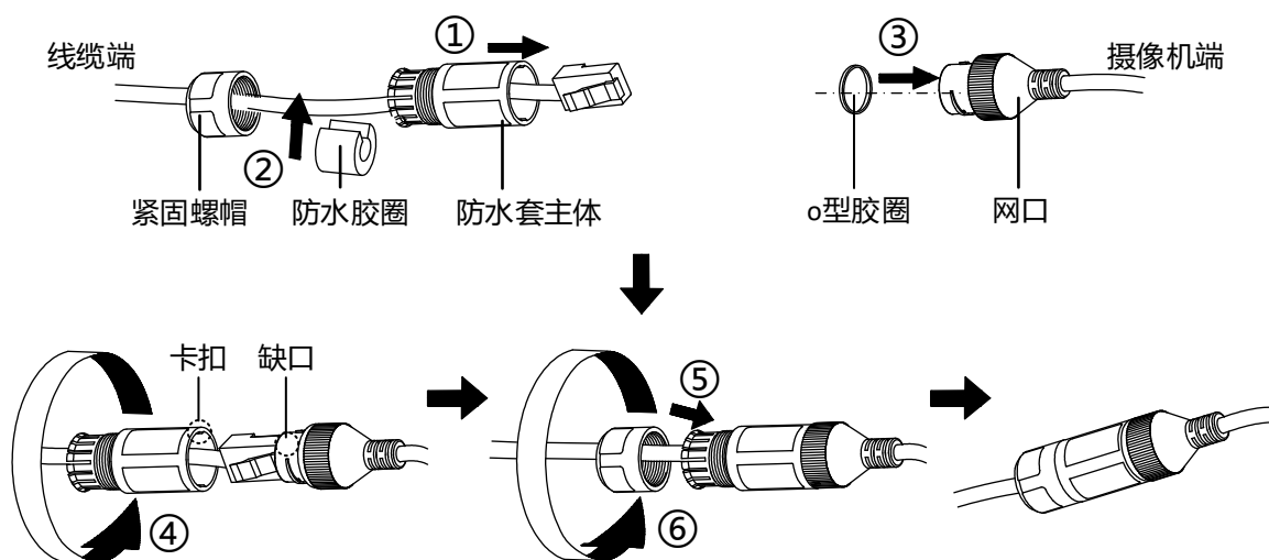
图1-11 安装网口防水套
