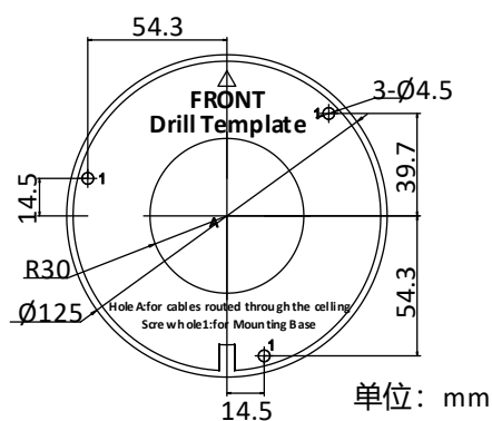
图1-3 安装孔位
