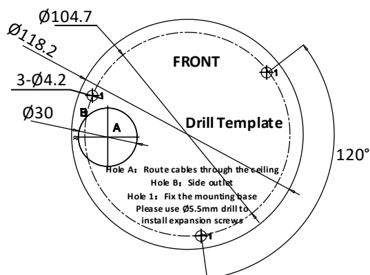
图1-8 安装孔位
